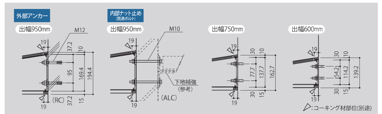
軒天部(ヒッコリー)
